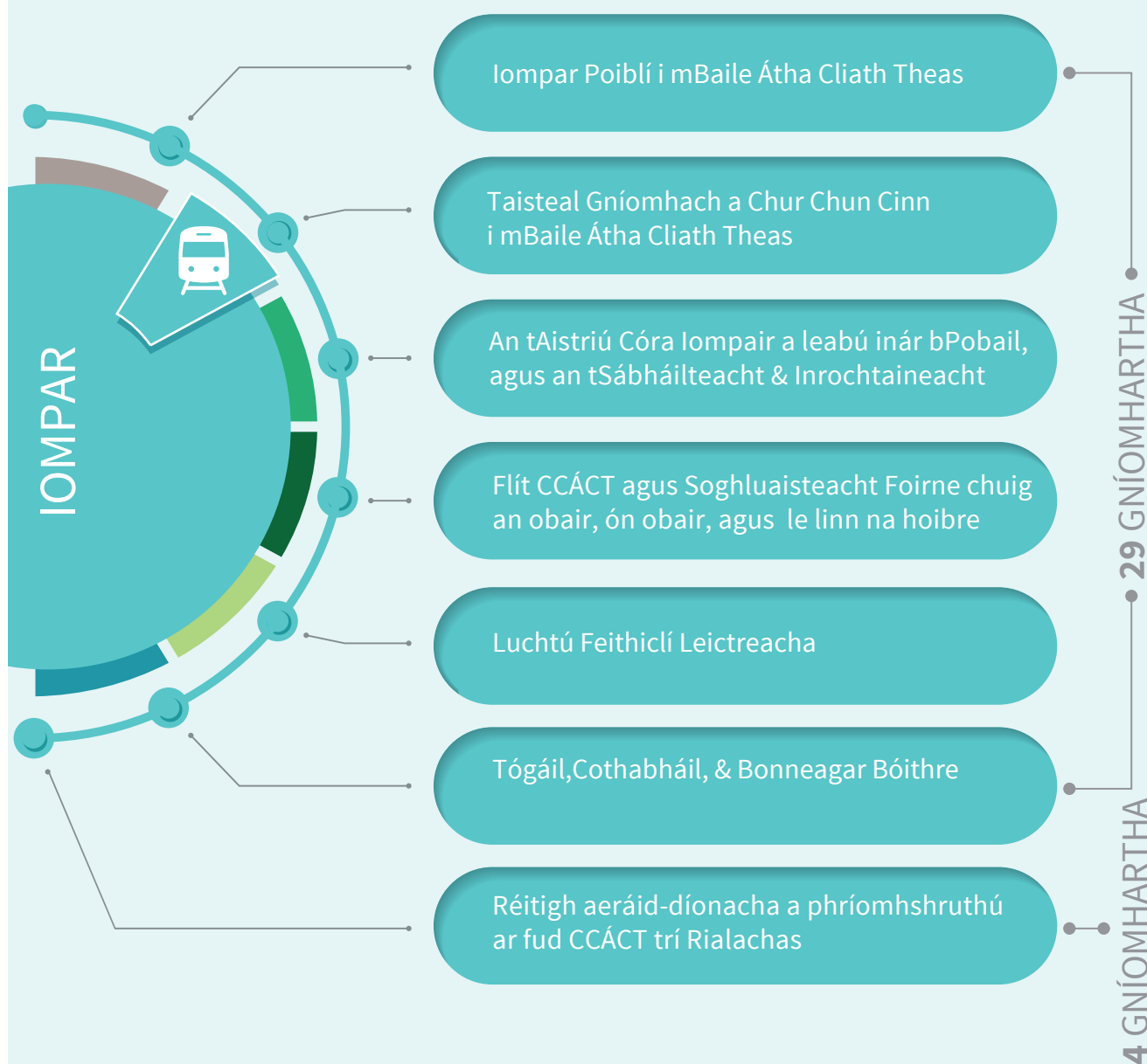
Fíor 5.2: Príomhréimsí Gníomhaithe CCÁCT chun aghaidh a thabhairt ar astaíochtaí a bhaineann le hiompar.
