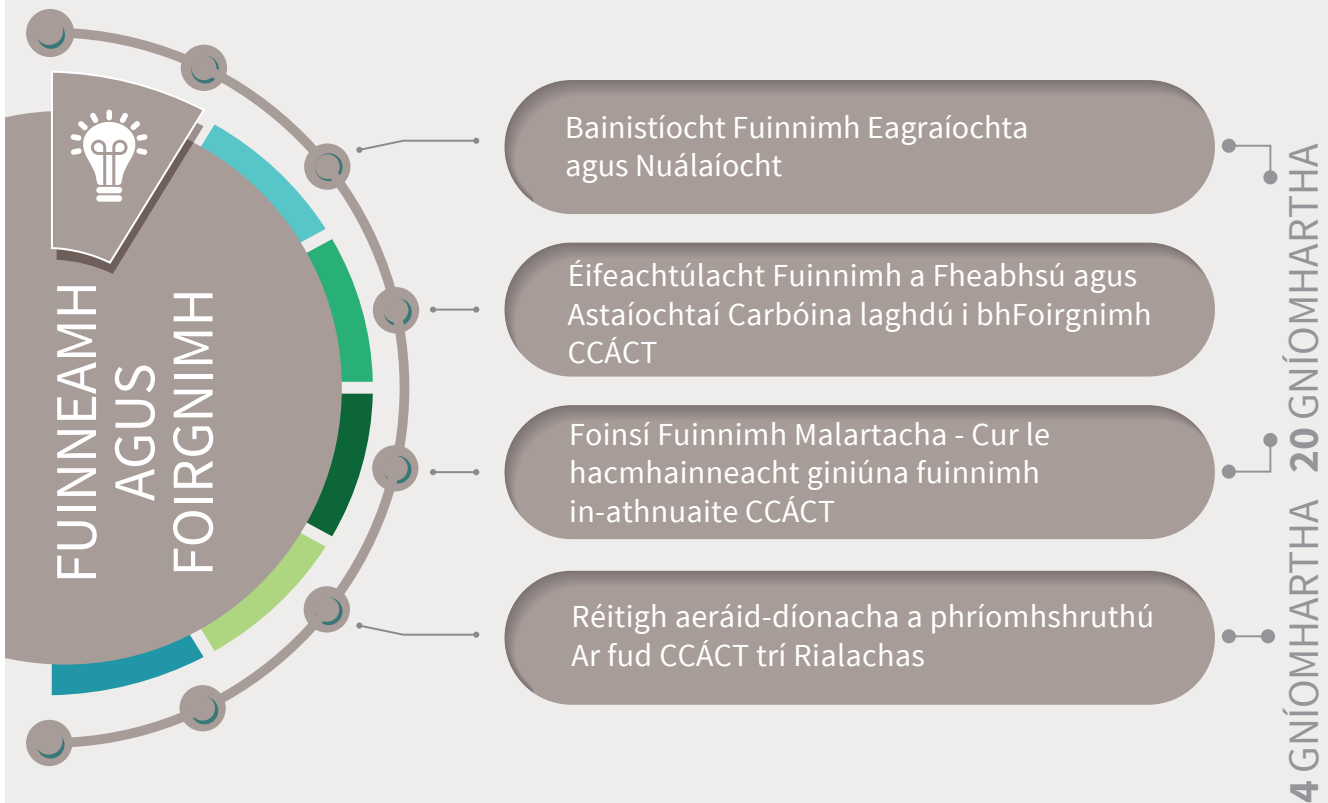
Fíor 5.1: Príomhréimsí Gníomhaithe CCÁCT d'Fhuinneamh agus d'Fhoirgnimh
