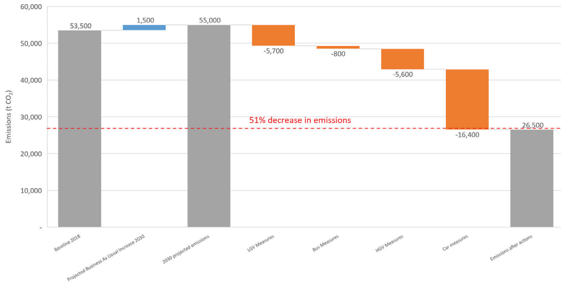
Fíor 6.13: Conair Aeráide Iompair DZ Chluain Dolcáin
