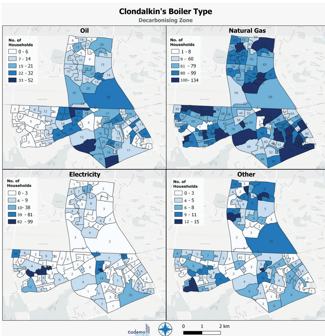
Fíor 6.7: Breosláí téimh a úsáideadh in aghaidh an cheantair bhig in DZ Chluain Dolcáin, de réir shonraí daonáirimh 2016.
