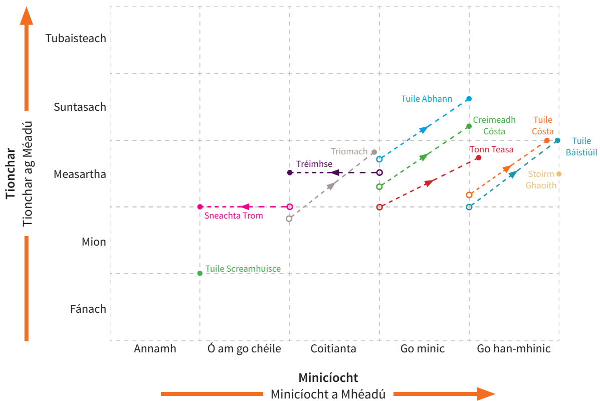
Fíor 3.9: Maitrís Riosca ag léiriú na n-athruithe riosca amach anseo i leith contúirtí a sainaitníodh laistigh de Bhaile Átha Cliath Theas. Do gach quais tá marcóir dlúth, a aithníonn an riosca don todhchaí, agus tá marcóir toll ann a léiríonn an riosca atá ann faoi láthair.
