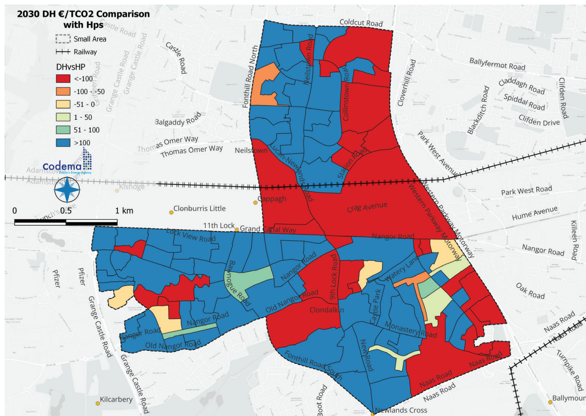
Fíor 6.16: Teaschaidéil agus téamh ceantair in DZ Chluain Dolcáin
