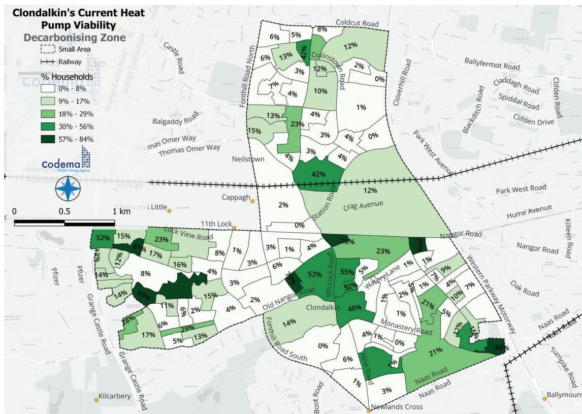
Fíor 6.15: Acmhainn oiriúnachta teaschaidéil in DZ Chluain Dolcáin
