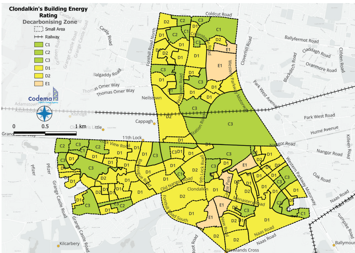
Fíor 6.6: Meánrátaí Fuinnimh Foirgnimh (RFF) Measta na dtithe i ngach ceantar beag laistigh de DZ Chluain Dolcáin
