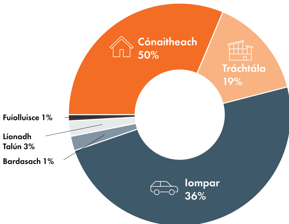
Fíor 6.4: Fardal maidir le hAstaíochtaí Bonnline (BEI) do Chriosanna Dícharbónaithe Chluain Dolcáin ag léiriú príomhfhoinsí d’astaíochtaí GCT
