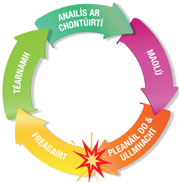
Fíor 4.1: An cur chuige i leith na Bainistíochta Móréigeandála
