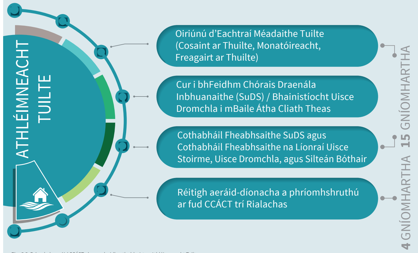
Fíor 5.5: Príomhchuspóirí CCÁCT chun aghaidh a thabhairt ar Athléimneacht Tuilte
