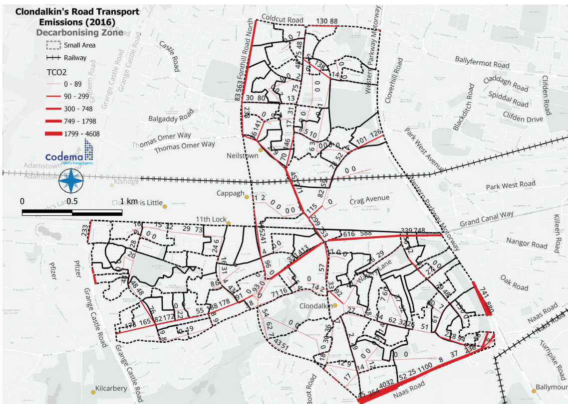
Fíor 6.9: Astaíochtaí ó thrácht ar bhóithre (tCO2) - arna fhorbairt bunaithe ar shonraí samhaltaithe curtha ar fáil ag an Údarás Náisiúnta Iompair (NTA)
