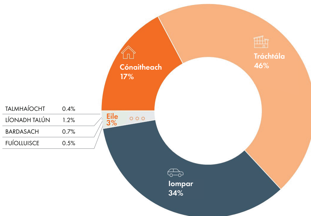
Fíor 3.4: Iomlán na nAstaíochtaí GCT do Bhaile Átha Cliath Theas de réir Earnála 2018 (%)
